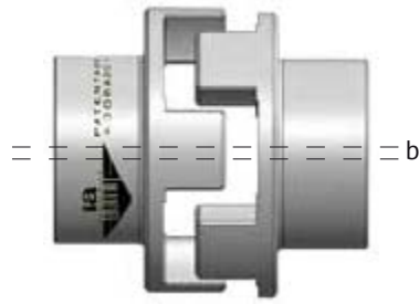
Desalineación RADIAL Radial misalignments / Désalignement Radial
