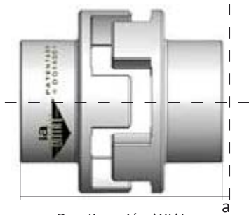
Desalineación AXIAL Axial misalignments / Désalignement axial
